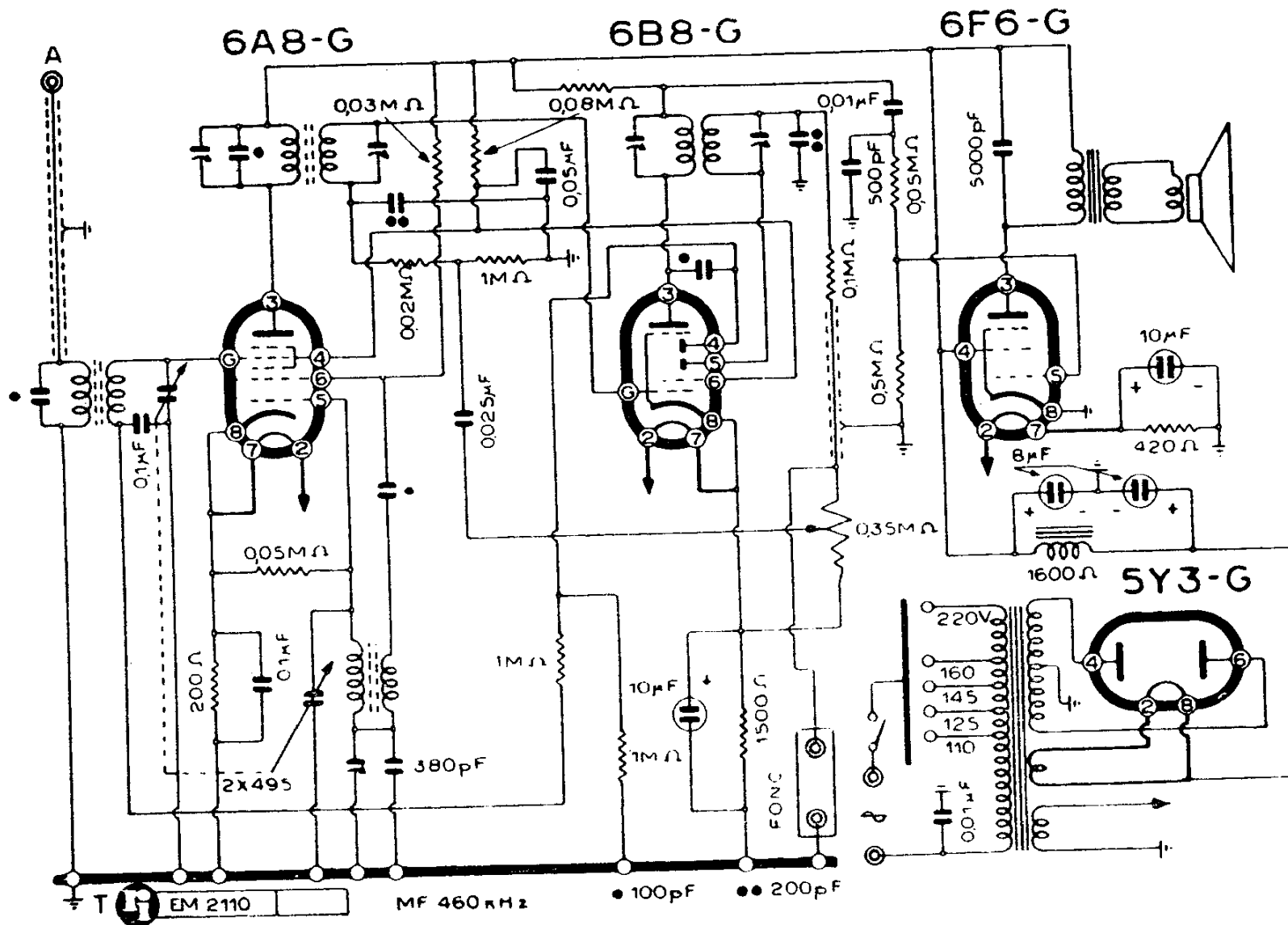
OFFICINE DI SAVIGLIANO - MOD. « 96 »
